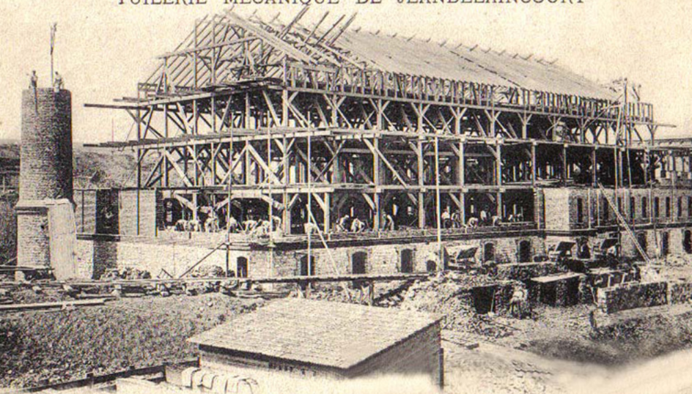
USINE III EN CONSTRUCTION - MAI 1912
